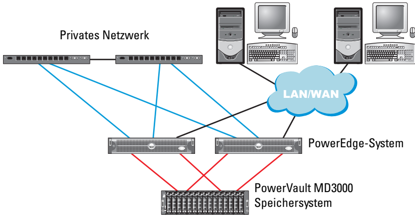
Abbildung 3. SAS-Cluster und PowerVault MD3000 verkabeln
